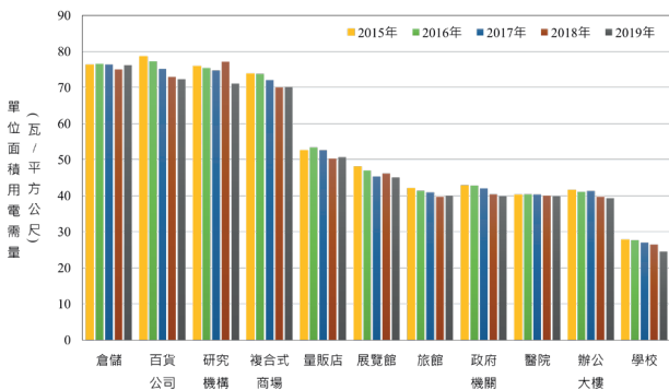
圖 8. 近五年單位面積耗電需量變化
