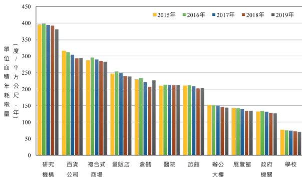
圖 7. 近五年單位面積年耗電量變化
